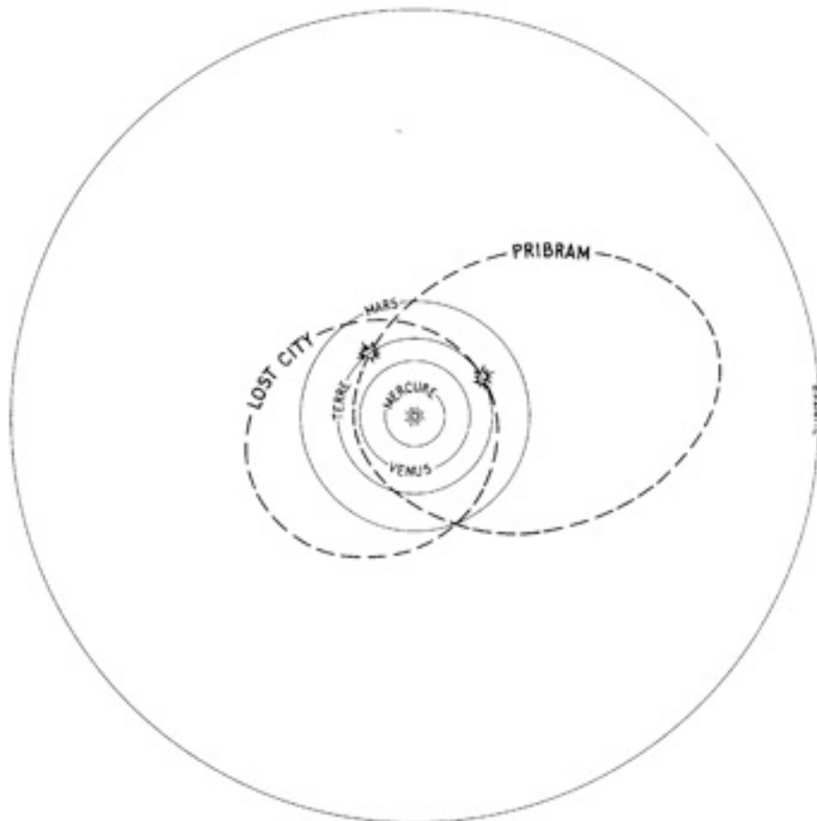
Reconstitution des orbites des météorites, Pribram et Lost-City, avant leur rencontre avec la Terre. La partie haute de ces orbites, l'apogée , se situe entre Mars et Jupiter, dans la zone des Astéroïdes
