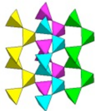
Spires hélicoïdales de tétraèdres SiO_4
