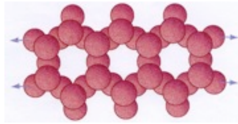
Si_4O_{11}
