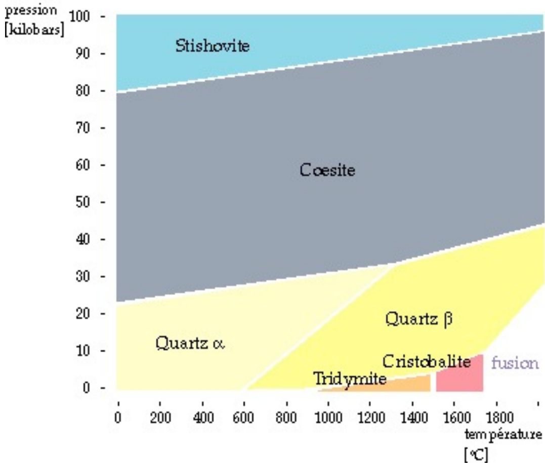
Diagramme d'équilibre de SiO 2 en fonction de la température et de la pression
