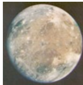
Ganymède , est le plus volumineux satellite du système solaire. Son rayon (5'262 km) est supérieur à celui de Mercure.
