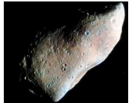
Gaspra, premier astéroïde survolé par la sonde spatiale Galileo en 1991.
