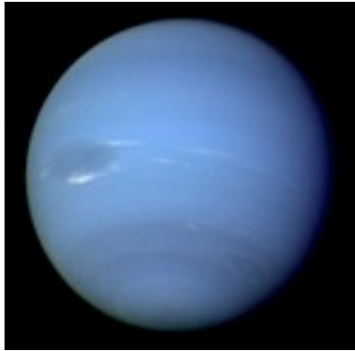
Neptune photographiée par la sonde Voyager 2 en 1989.
