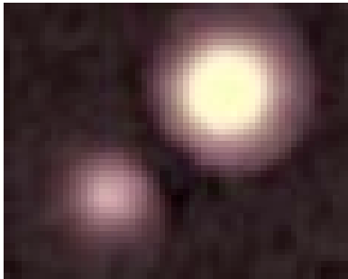
Pluton et son satellite Charon
