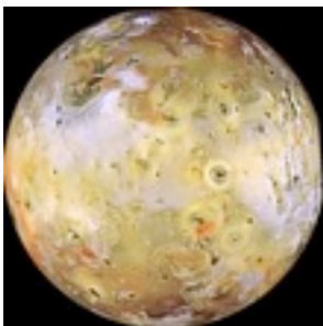
Io , dont le diamètre est de 3720 km, est remarquable par les éruptions volcaniques qu'on y a observées.
