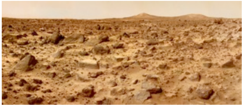
Aspect de la surface de Mars
