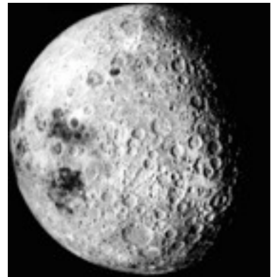
Face cachée cartographiée par Appolo 16 en 1972
