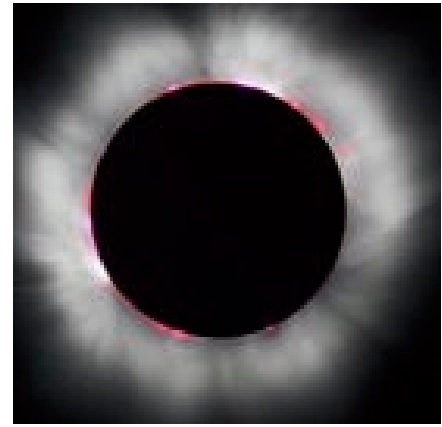
Couronne (en rouge) et chromosphère (en gris) photographées lors de l'éclipse totale du 11 août 1999 (Wikipedia)
