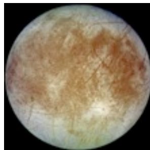
Europa , de taille comparable à la Lune, est parfaitement lisse. Sa composition est analogue à celle des météorites pierreuses
